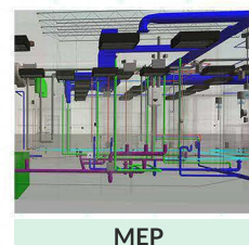
MEP
